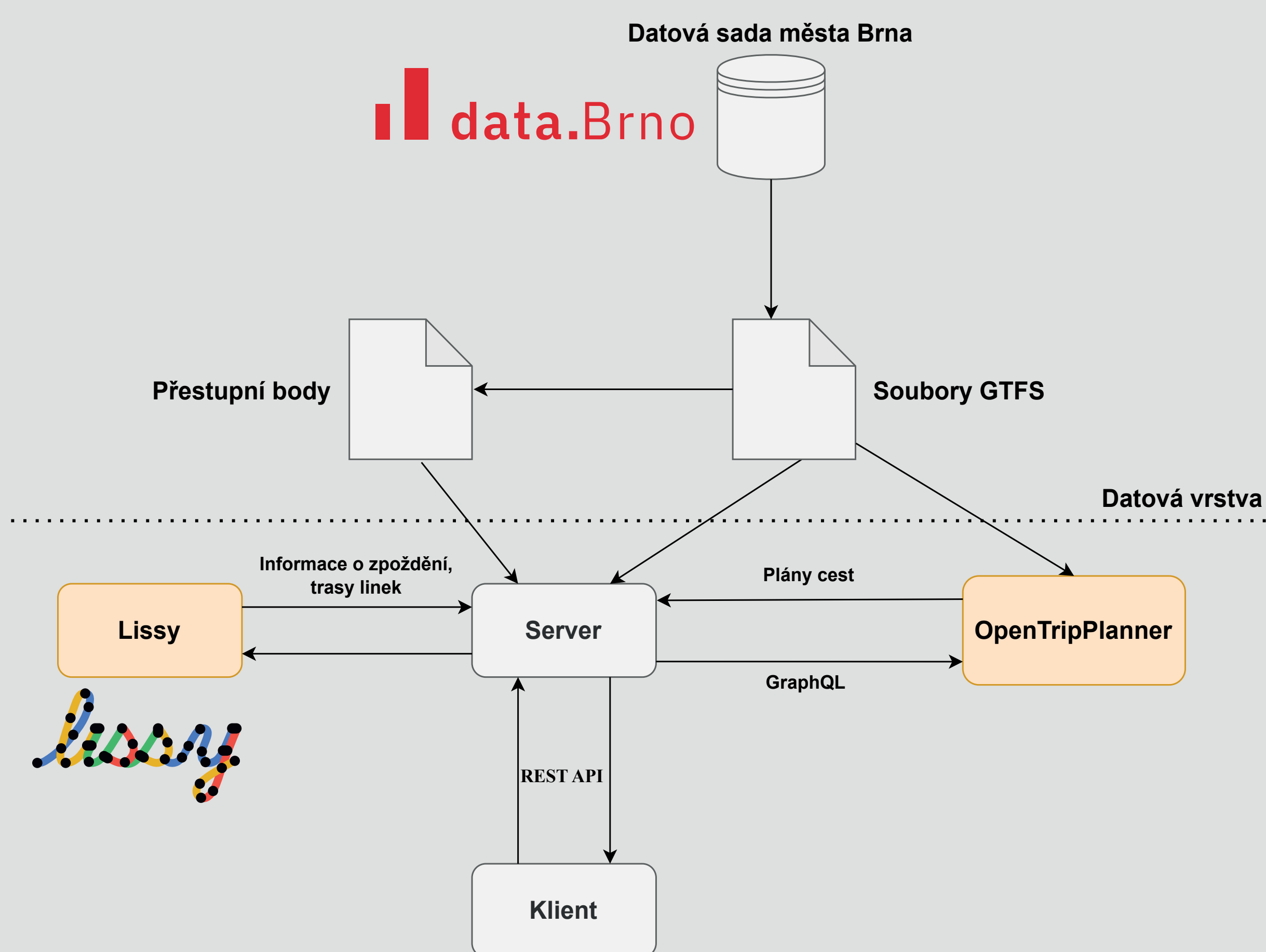
Architektura aplikace (1)
